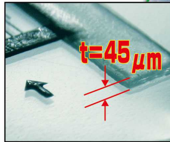
□メッシュ：250-30 3D □乳剤：NU-30(汎用・厚膜用乳剤) □乳剤厚：+20μm
